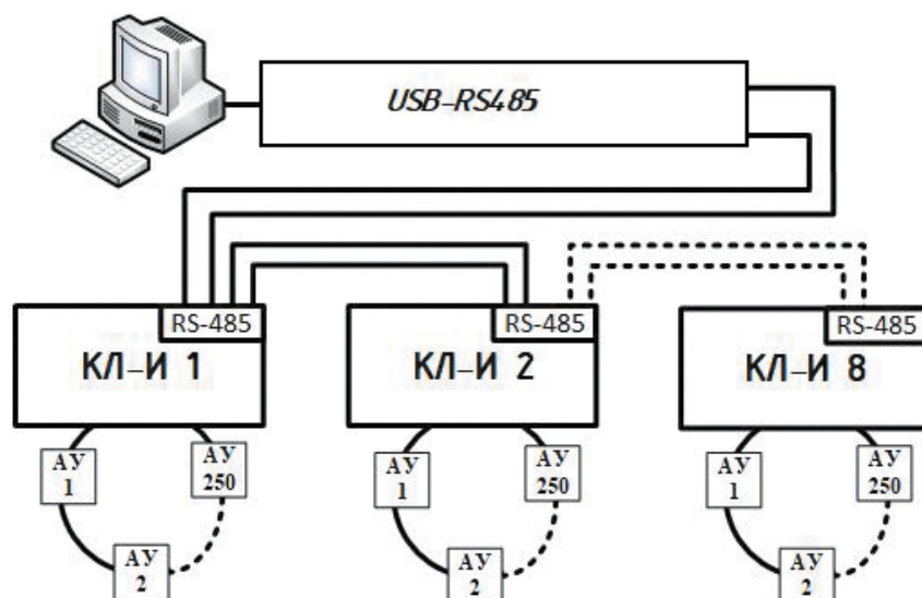
Схема подключения
